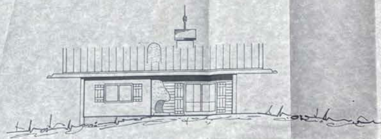
westansicht
