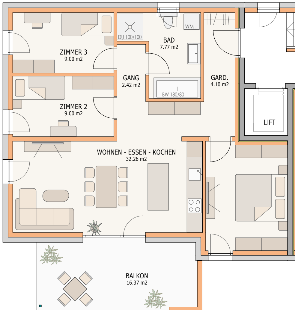
OBERGESCHOSS TOP A-02 WNF (Wohnnutzfläche) ca. 77.56 m 2
