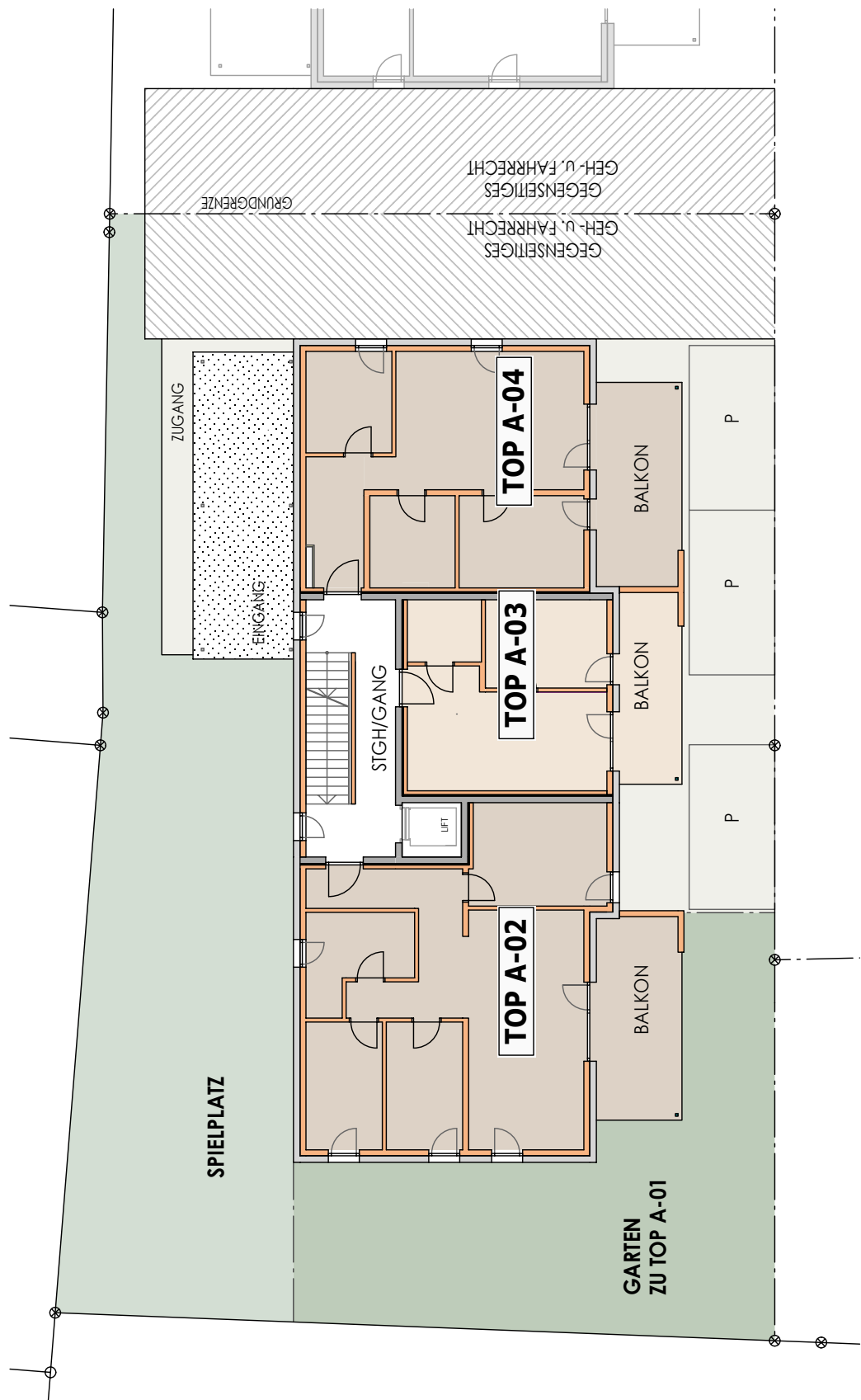
LAGEPLAN OBERGESCHOSS
