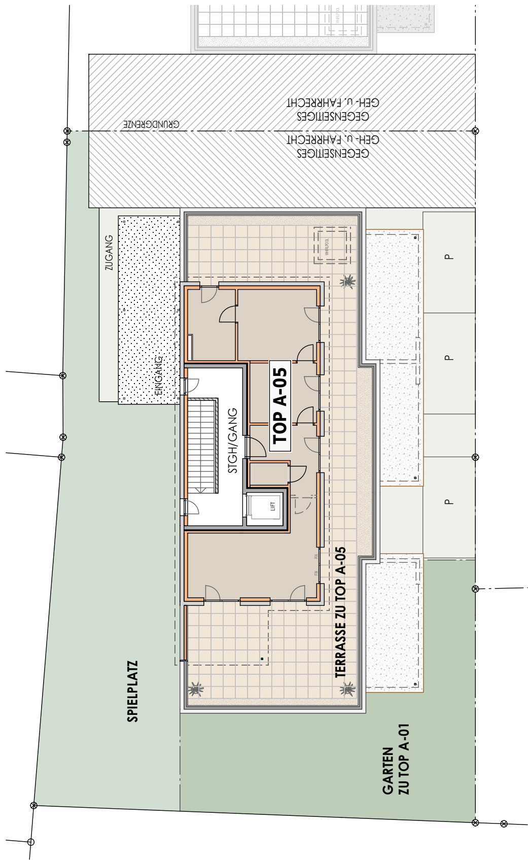
LAGEPLAN DACHGESCHOSS
