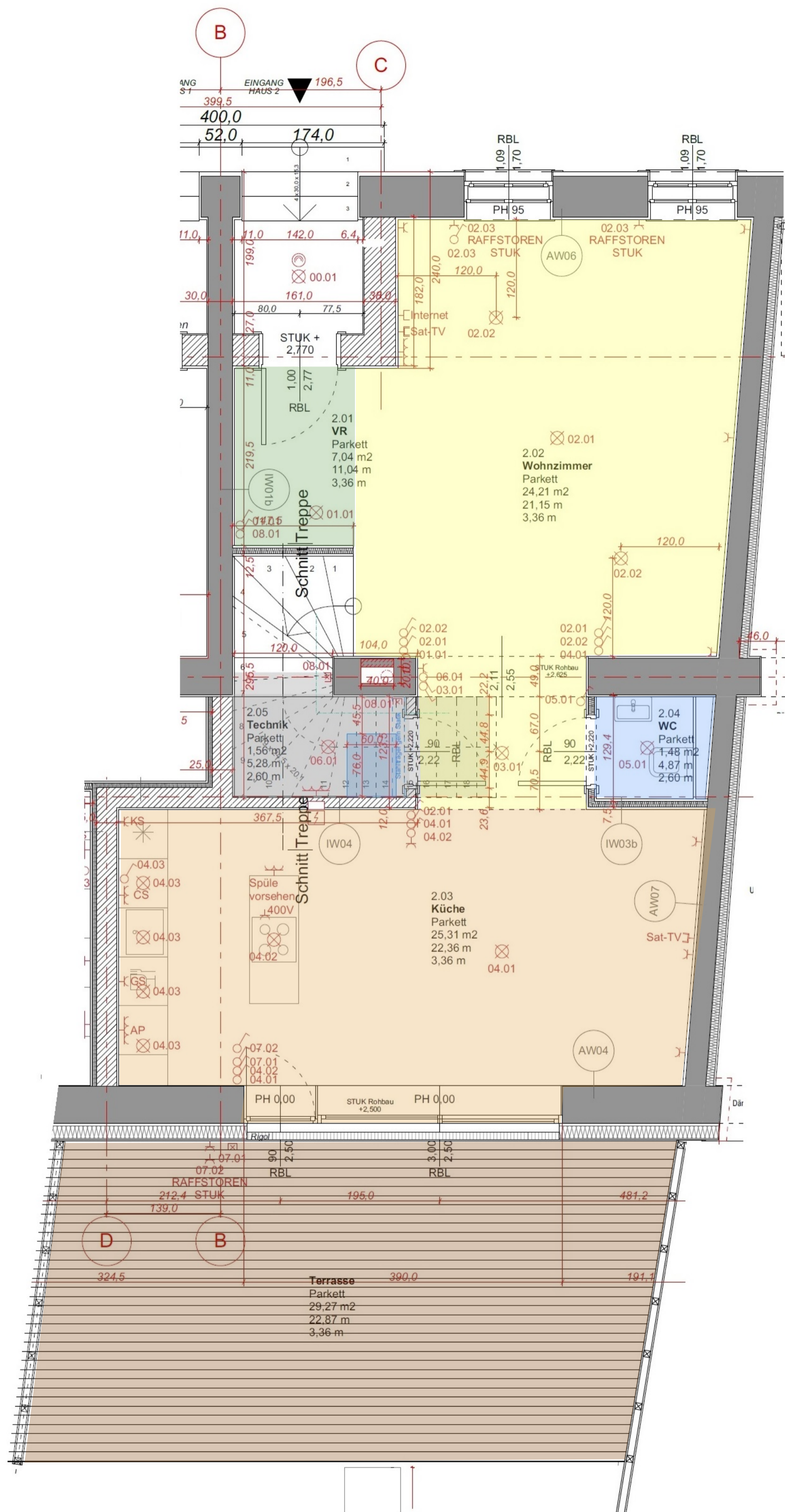
ERDGESCHOSS
