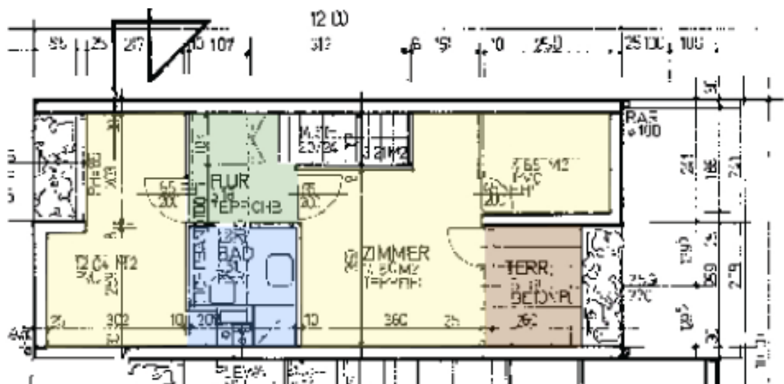
2.OG
