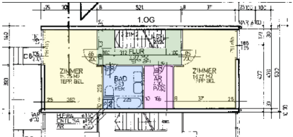
1.OG
