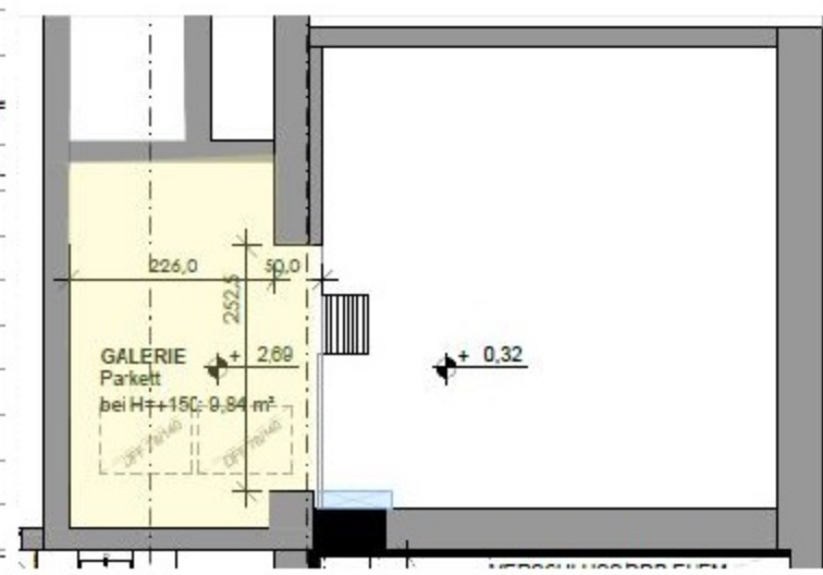
GRUNDRISS DG2
