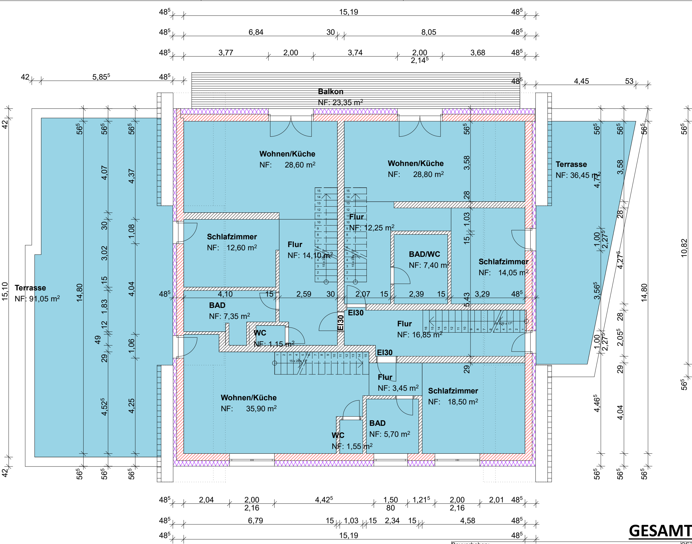
GRUNDRISS 1. OBERGESCHOSS
