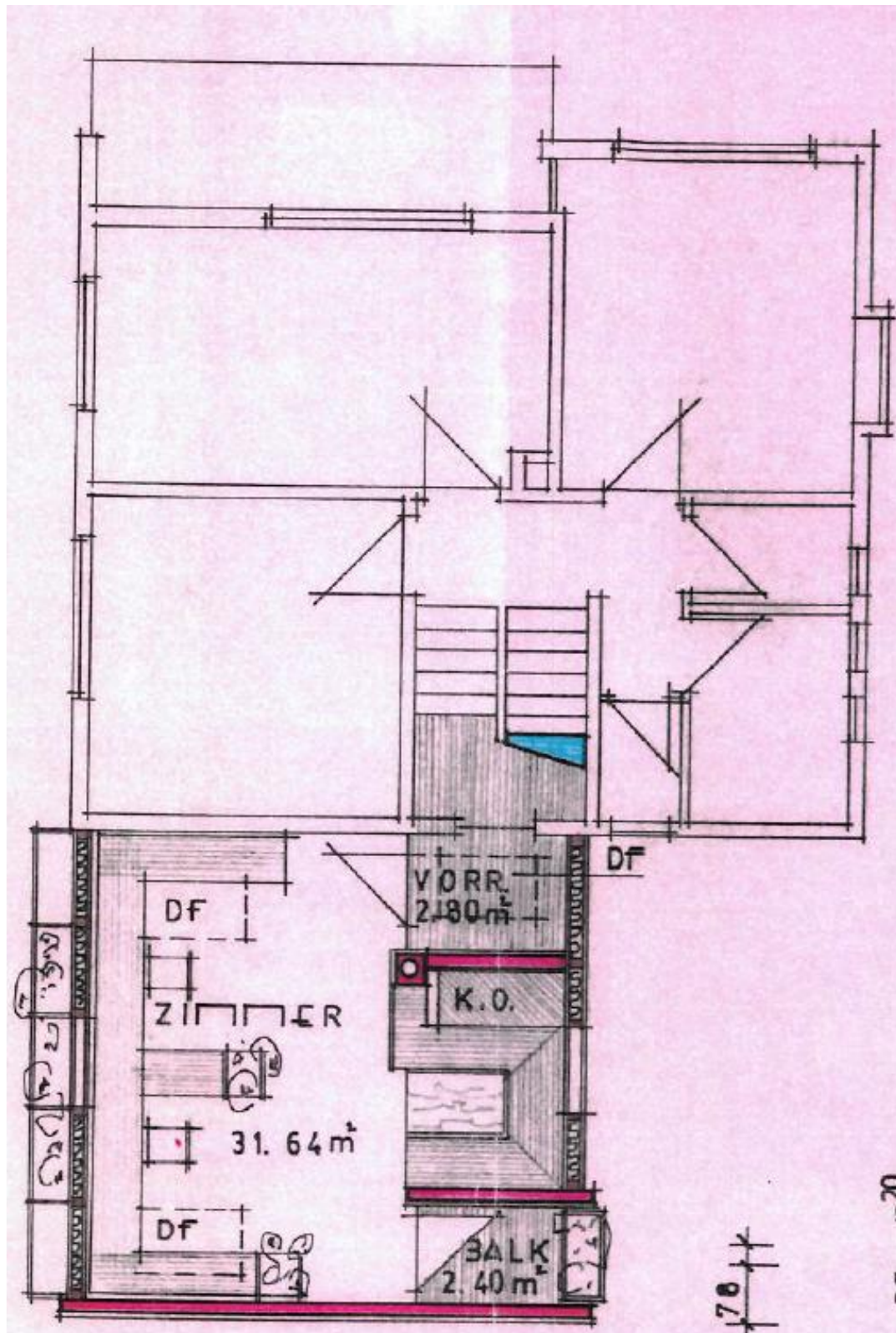
Grundriss Zwischengeschoß
