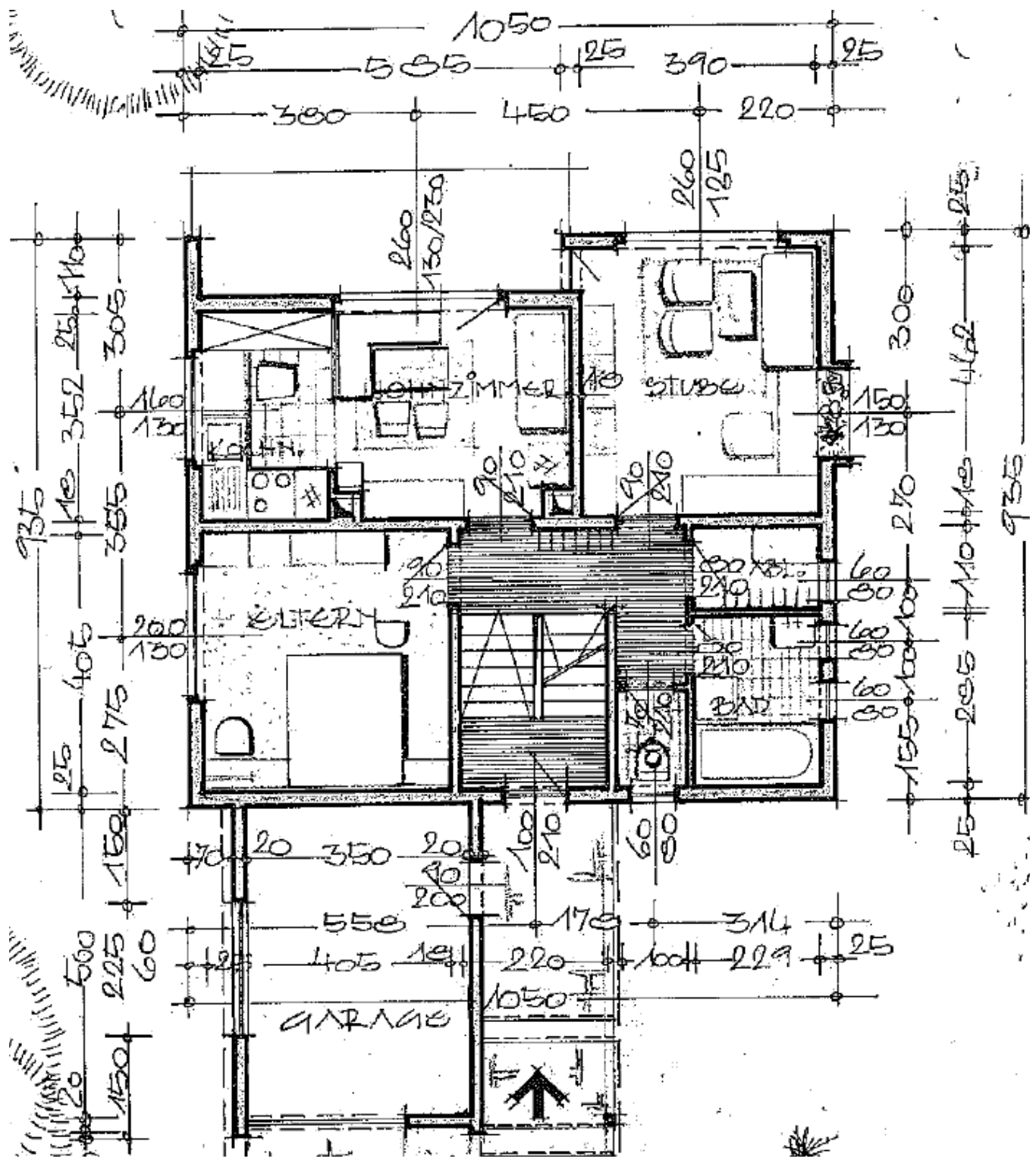
Grundriss Erdgeschoß
