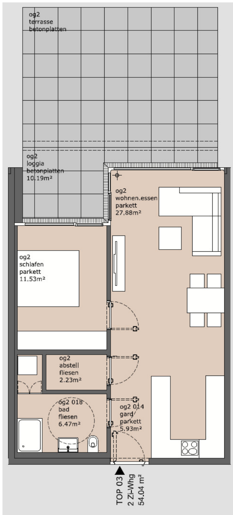
Grundriss Top 3
