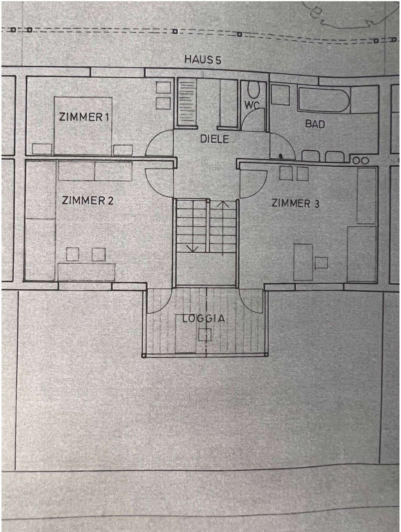
Obergeschoß
