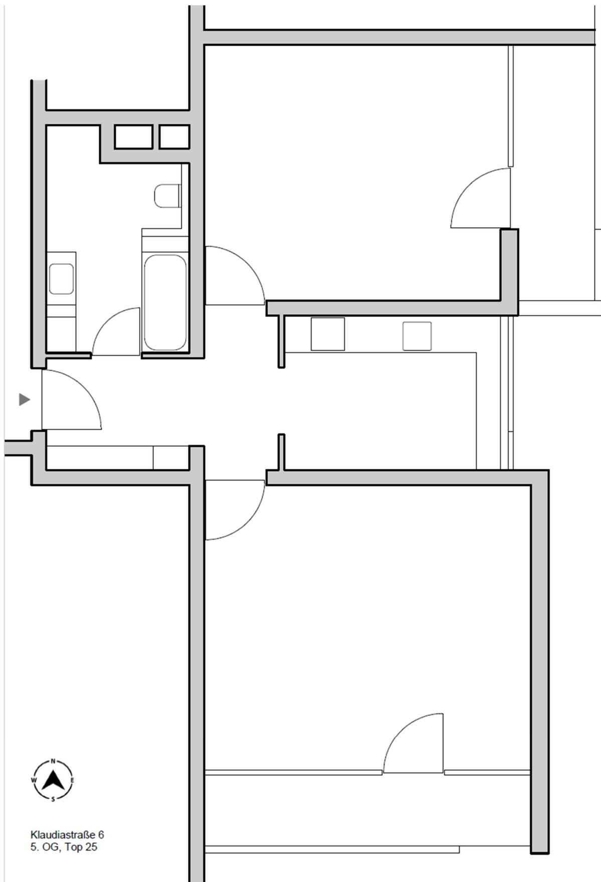
Grundriss
