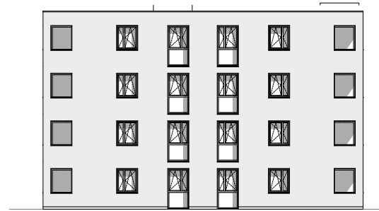
Ansicht Süd-Ost
