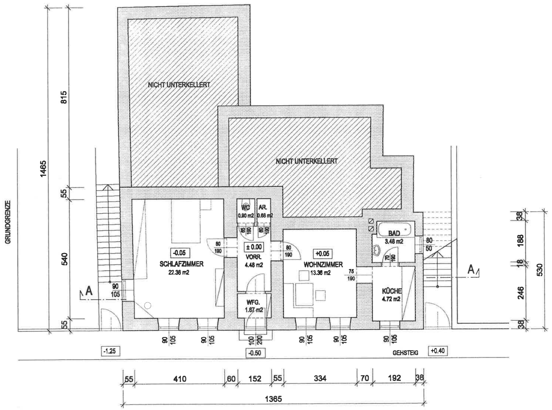
ERDGESCHOSS
