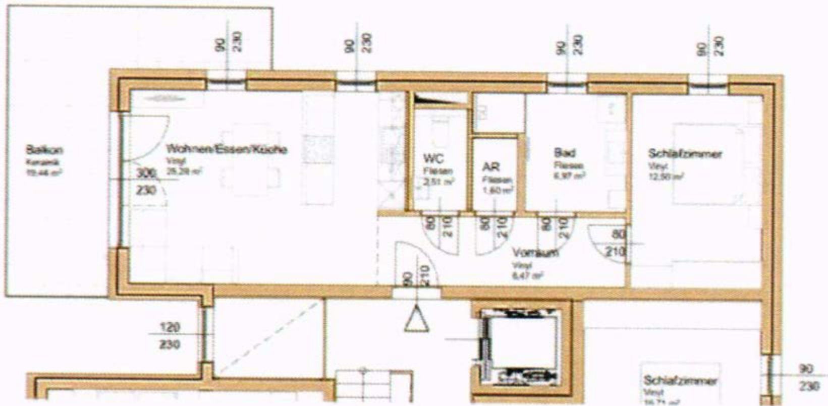
GRUNDRISS HAUS D TOP 4
